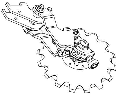
72455040 - C.J. TAPADOR DE SULCOS ESQUERDO
