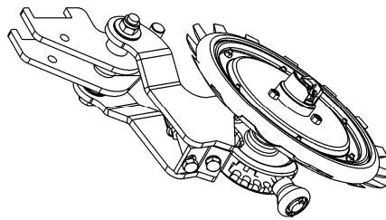
72455041 - C.J. TAPADOR DE SULCOS DIREITO
